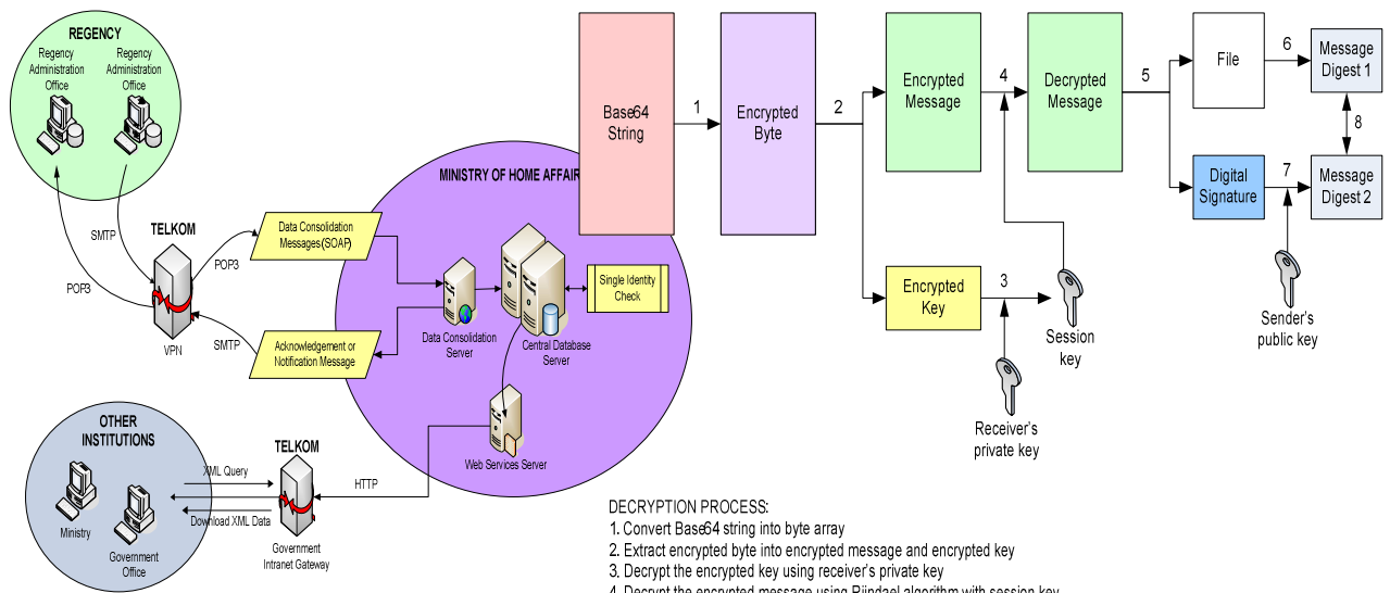
Gambar 7. Arsitektur Jaringan
